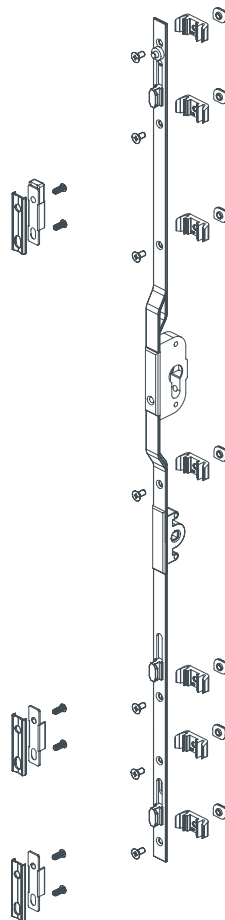
Serratura multipunto con cilindro e maniglia vista interna apertura laterale
