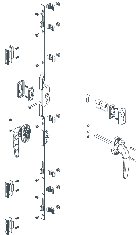
Serratura multipunto con doppio cilindro e doppia maniglia vista interna apertura laterale
